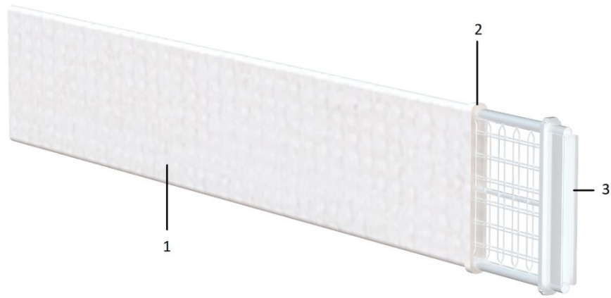
1 Filtrační kapsa 2 Těsnící manžeta 3 Rám filtrační kapsy
