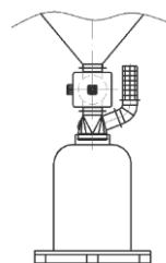
Rotační podavač a BIG-BAG
