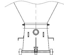
Šnek, rotační podavač a BIG-BAG
