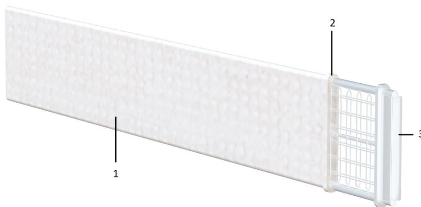
1 Filtrační kapsa 2 Těsnící manžeta 3 Rám filtrační kapsy
